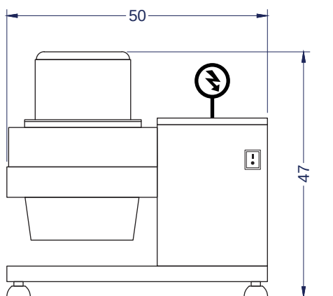
Vista Elevación
